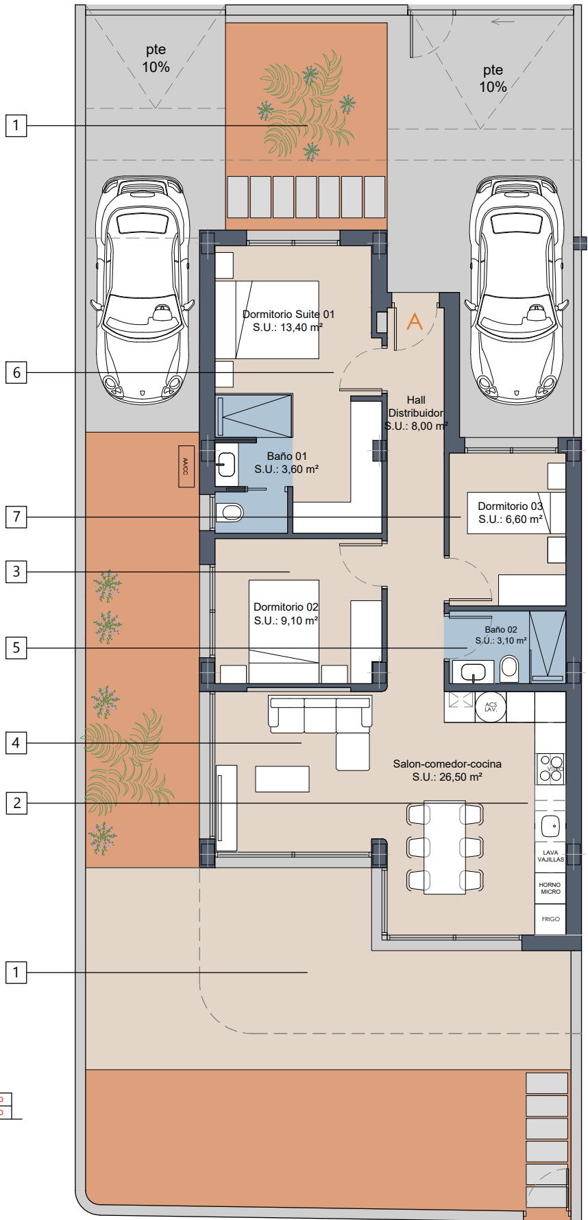
PLANTA BAJA
